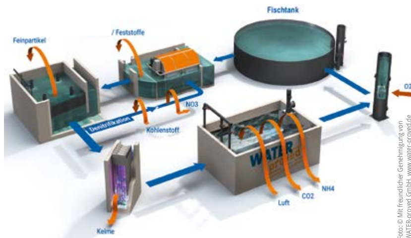
Schema einer Kreislaufanlage zur Fischzucht – Das Wasser wird mechanisch und biologisch gereinigt, desinfiziert, mit Sauerstoff angereichert und wieder in die Fischbecken geleitet.
