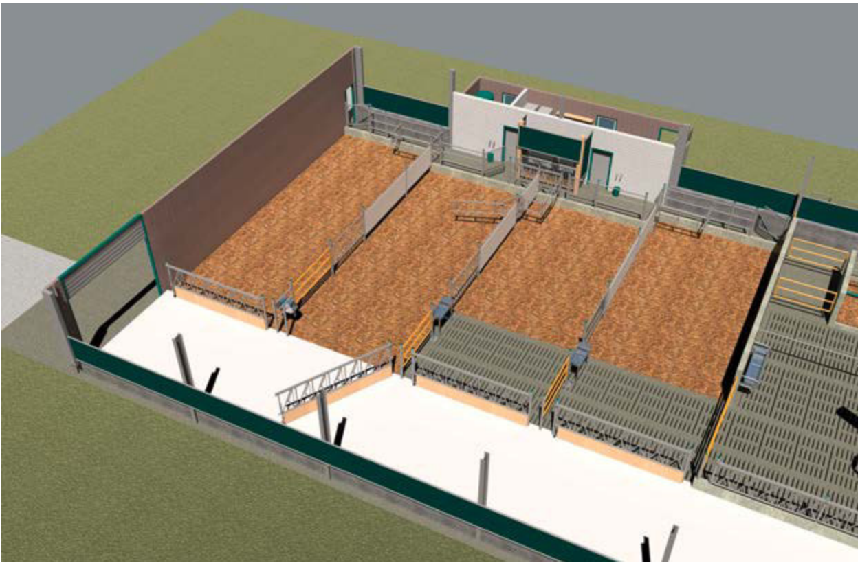
Einflächenbuchten mit Stroh (links) sowie Zweiflächenbucht mit Stroh und Spalten (rechts).
