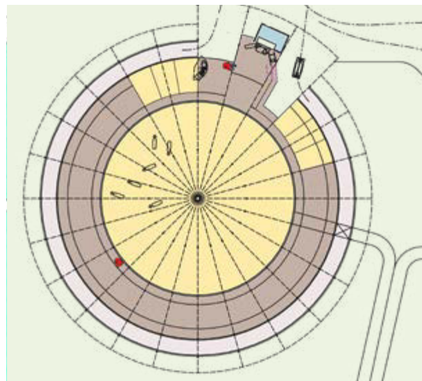
Ein Abteil des „Tierwohlstalles“ für 60 Kühe.
