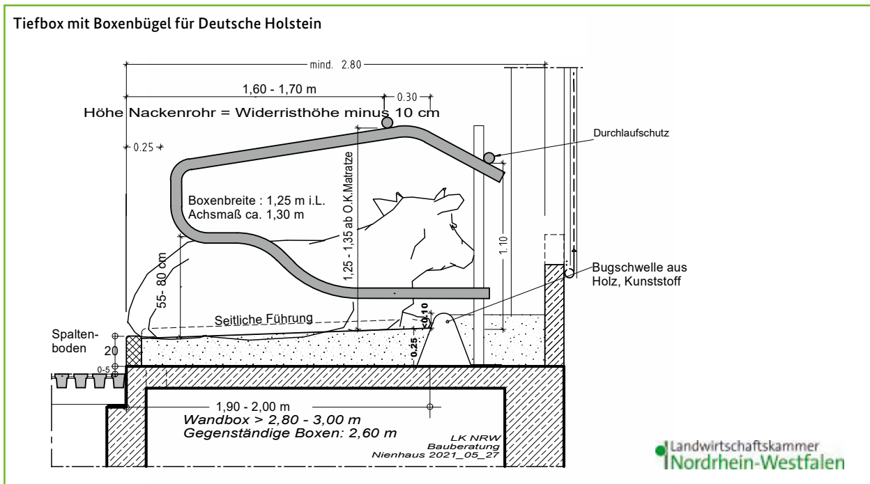
Schemazeichnung einer Tiefbox.
