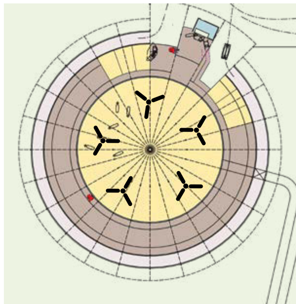
Lüftungssystem im Roundhouse.
