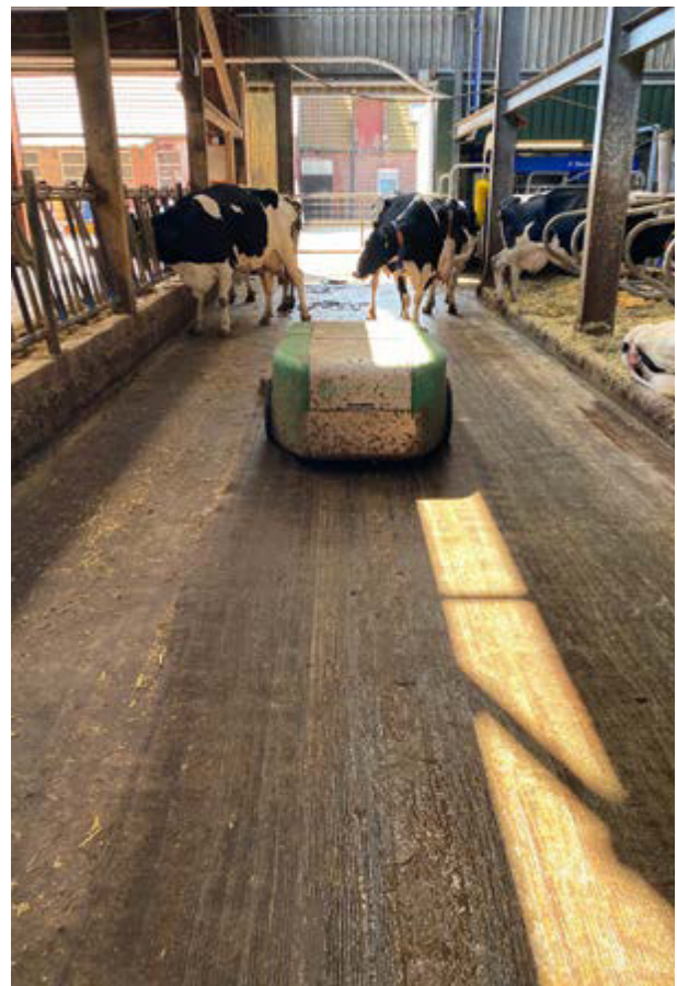
Güllekollektoren nehmen die Gülle von der Lauffläche auf und reduzieren dadurch die Emissionen.
