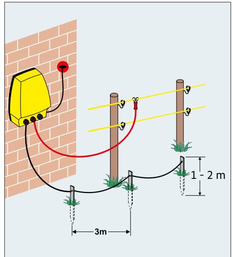
Abbildung 2: Weidezaungerät mit Netzanschluss.
