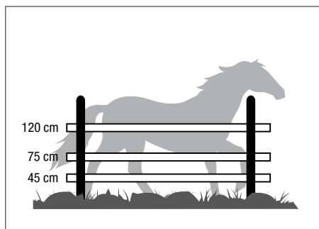
Abbildung 14: Zaunhöhen für Kleinpferde.
